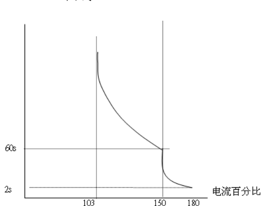
403 OL1 曲线
