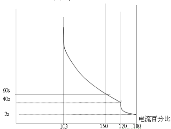
401 402 OL1 曲线
